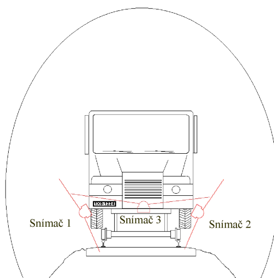
Obr. 9: Možné osazení drezíny MD1 snímači profilu
