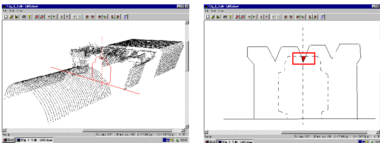
Obr. 12: Kontrola průjezdného profilu
