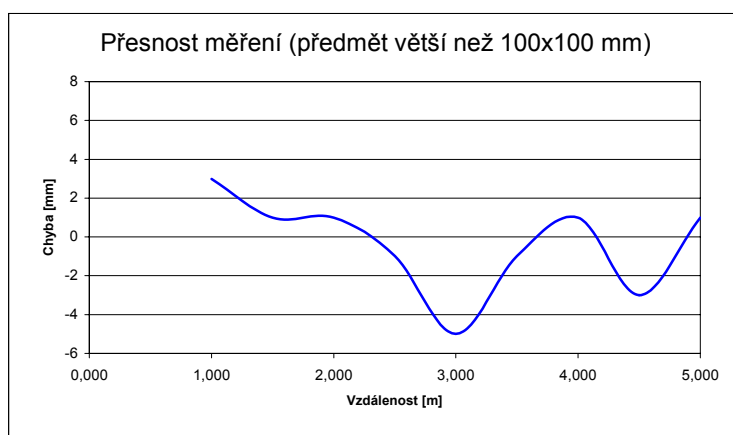
Obr. 4: Přesnost měření
