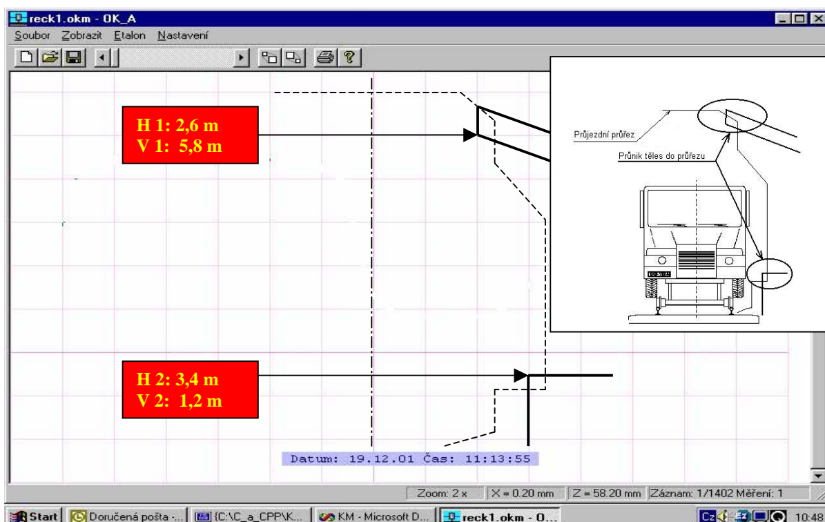
Obr. 10: Měření profilu nástupiště a vykreslení průniku do definovaného profilu
