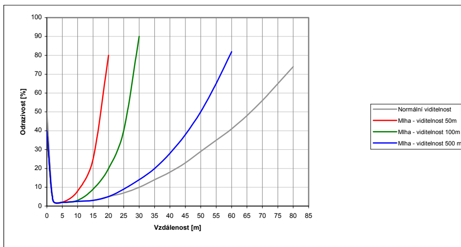
Obr. 1: Závislost vzdálenosti na prostředí a odrazivosti
