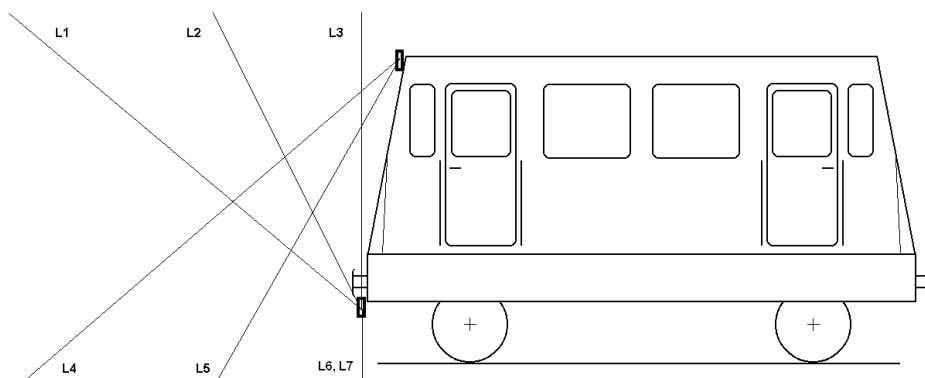
Obr. 8: Možnost umístění laserových snímačů
